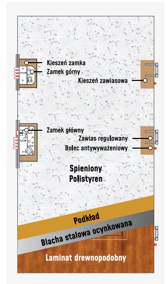
PROFIL SKRZYDŁA NORMAL
