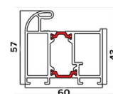
Rysunek techniczny
