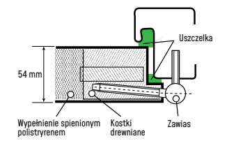
PROFIL SKRZYDŁA NORMAL
