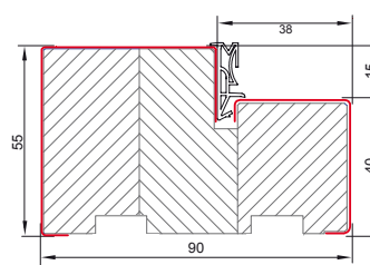
ościeżnica stalowo-drewniana (za dopłatą)
