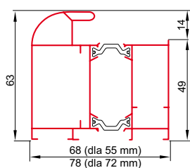
ościeżnica aluminiowa z przegrodą termiczną
