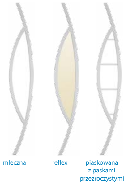
Przeszklenia S40 – ramka INOX
