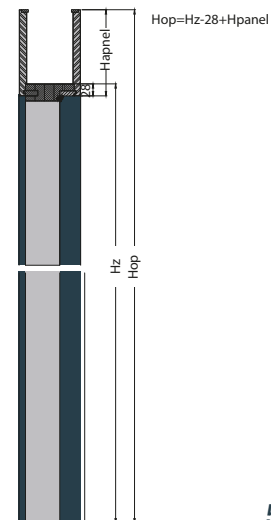
OŚCIEŻNICA Z PANELEM
