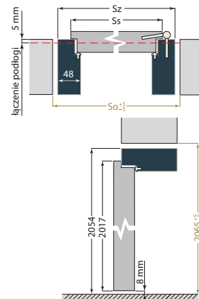
OŚCIEŻNICA STAŁA OPASKI 60/75mm (skrzydło przylgowe)
