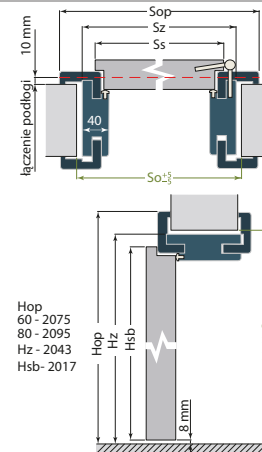
OŚCIEŻNICA Z PANELEM
