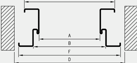
przekrój poprzeczny
