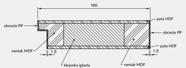
PRZEKRÓJ RAMIĄKA PIONOWEGO
