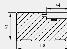
Przekrój poziomy ościeżnicy w murze
