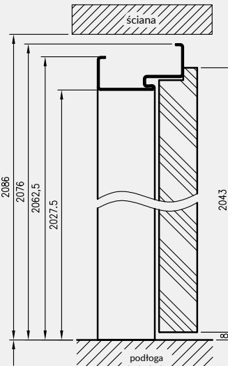
przekrój poprzeczny alternatywny sposób montażu
