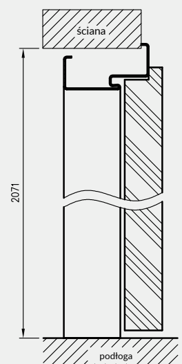
przekrój pionowy alternatywny sposób montażu
